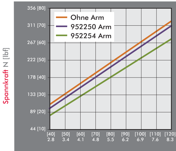
Serie 9522 Kolbenkraft
