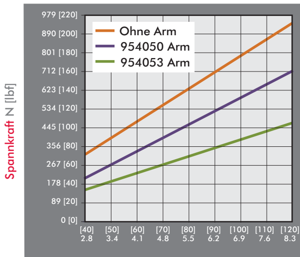
Serie 9530 Kolbenkraft
