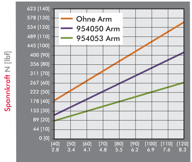
Serie 9540 Kolbenkraft
